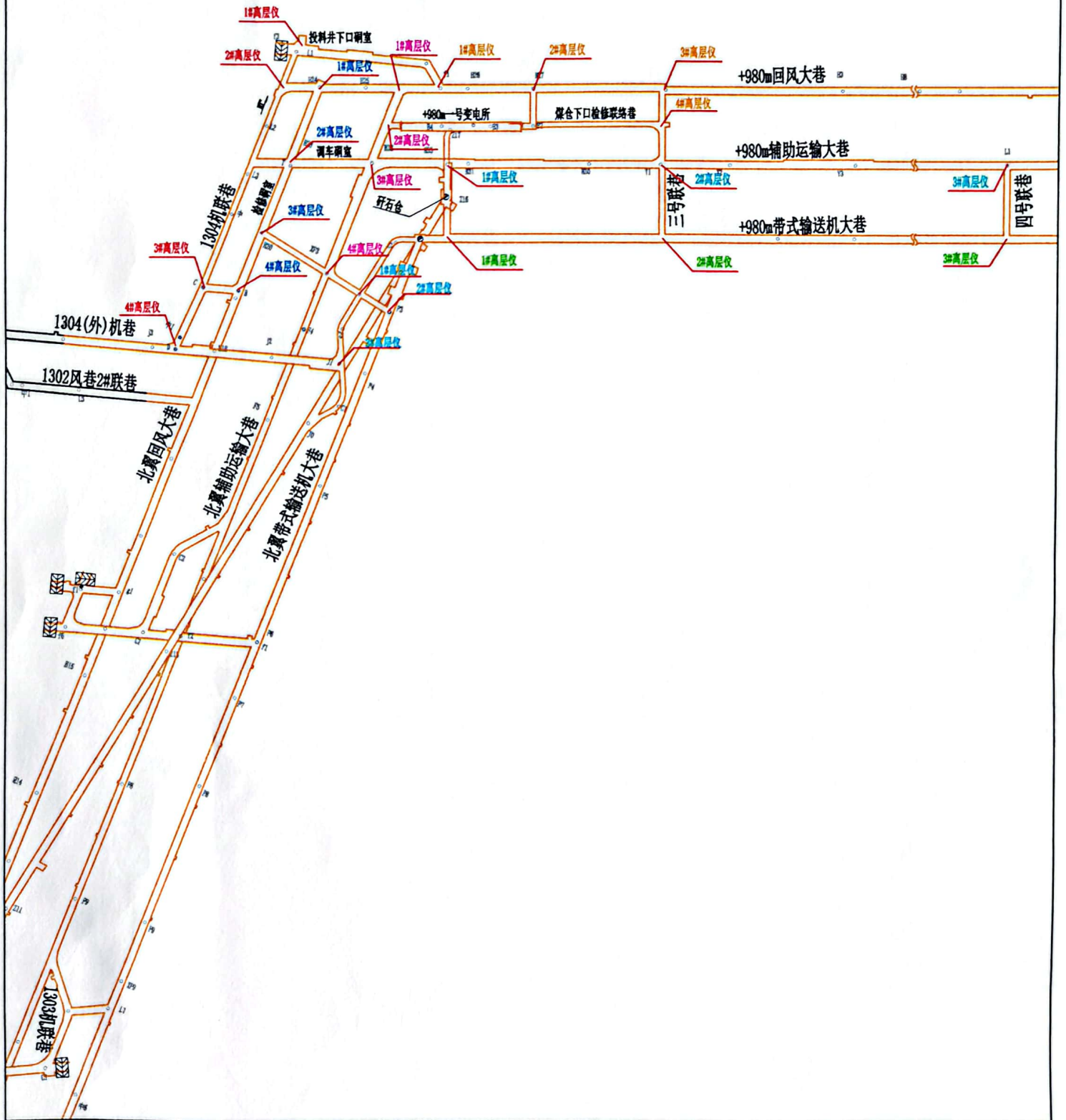
附图1：顶板离层仪平面布置图
